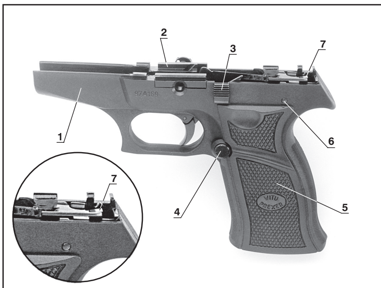
Fot. 4 Zmontowany szkielet WIST 94: 1 - szkielet; 2 - mechanizm spustowy; 3 - zaczep zamka; 4 - zatrzask magazynka; 5 - okładka lewa; 6 - oś wkładki tylnej; 7 - zaczep szyny spustowej (integralna część szyny spustowej)
