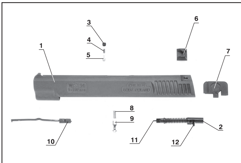
Fot. 8 Zamek całkowicie rozłożony: 1 - zamek; 2 - zespół iglicy; 3 - wkrętka; 4 - sprężyna wskaźnika naboju; 5 - wskaźnik naboju; 6 - szczyrbinka; 7 - zastawka; 8 - sprężyna blokady; 9 - blokada iglicy; 10 - wyciąg; 11 - grot iglicy i 12 - zaczep iglicy (integralne części iglicy)
